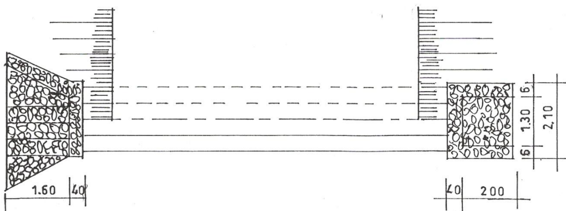
COUPE AA 4.0 1.05 4.0 1.85
